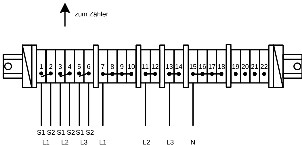
A 1.02 Klemmenleiste für den Einsatz auf Wechselftafeln sowie im Zählerfeld
